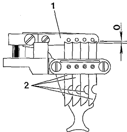
DETT. A
